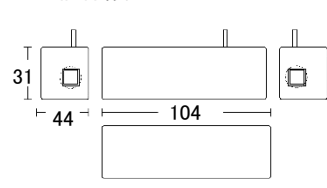
概観寸法 mm (通信保護モジュール)
