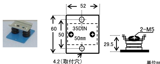
絶縁タイプ取付ベース(MK506J)使用例
