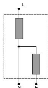
回路図
